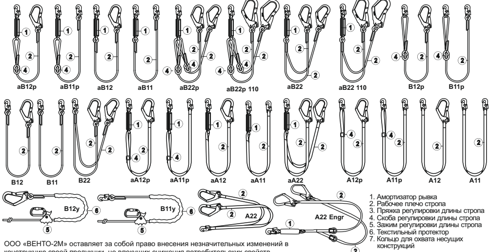
Рис. 3. Внешний вид, состав стропов
