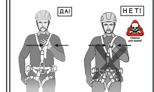
Рис. 11. Соединительно-амортизирующая подсистема
