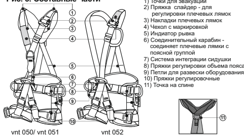
Рис. 3. Составные части
