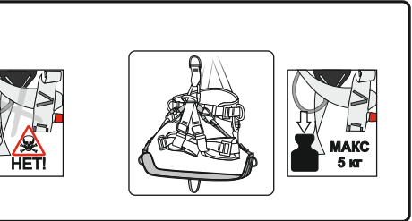
Рис. 16. Способ интеграции рабочего сиденья
