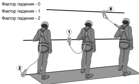
Рис. 4. Графическая схема к определению фактора падения
