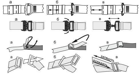
Рис. 5. Типы используемых пряжек, способы заправки
