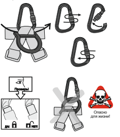
Рис. 10. Страховочная система
